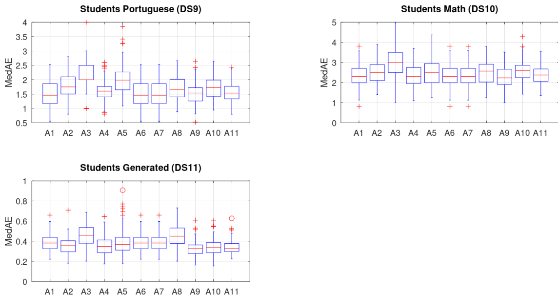
FIGURE 6.14 – Erreurs médianes absolues (MAE - Median Absolute Error) obtenues pour les dix algorithmes testés sur les jeux de données DS9, DS10 et DS11.
