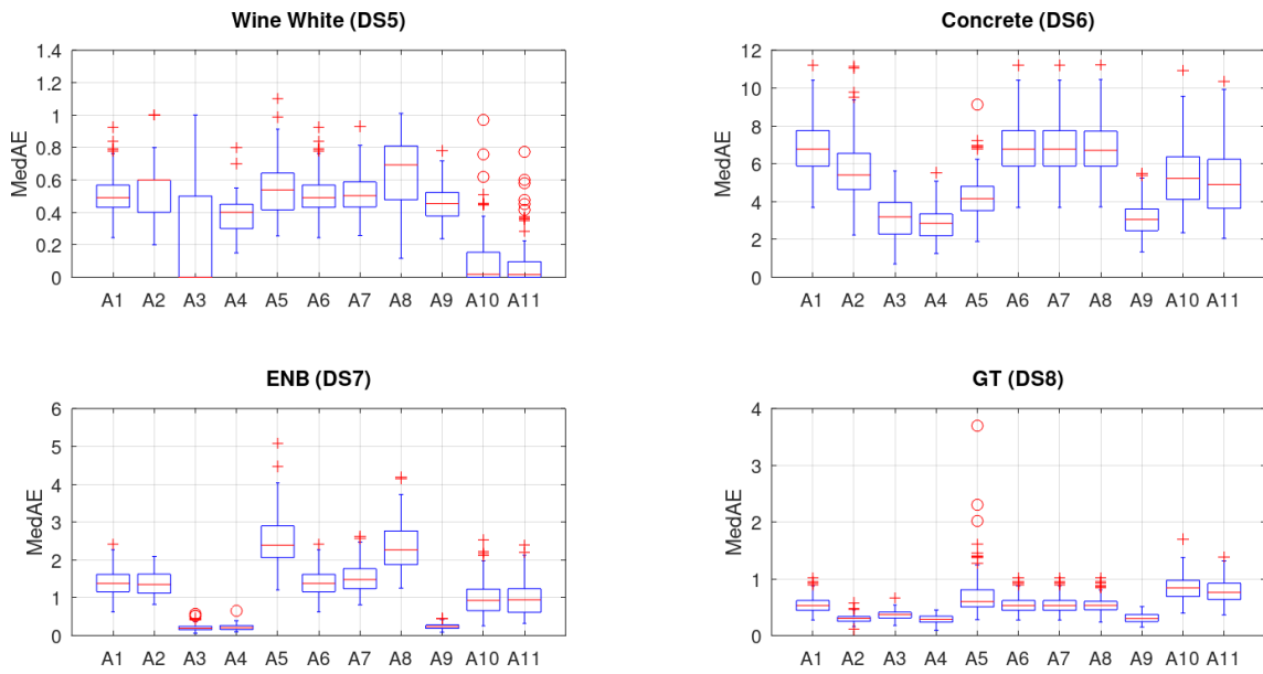
FIGURE 6.13 – Erreurs médianes absolues (MAE - Median Absolute Error) obtenues pour les dix algorithmes testés sur les jeux de données DS5, DS6, DS7 et DS8.
