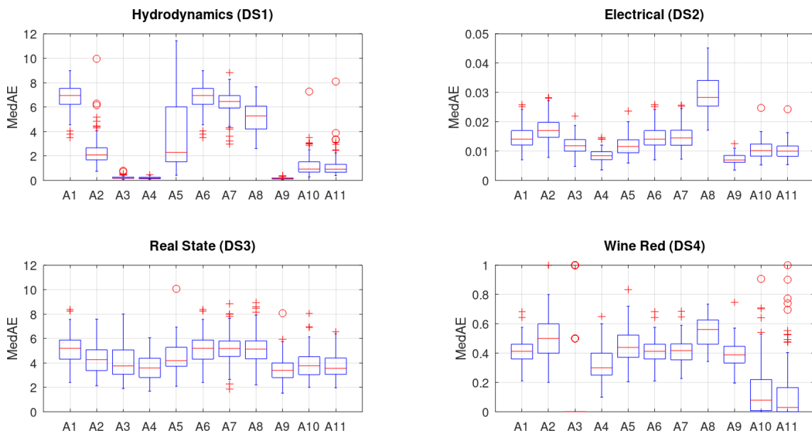
FIGURE 6.12 – Erreurs médianes absolues (MAE - Median Absolute Error) obtenues pour les dix algorithmes testés sur les jeux de données DS1, DS2, DS3 et DS4.
