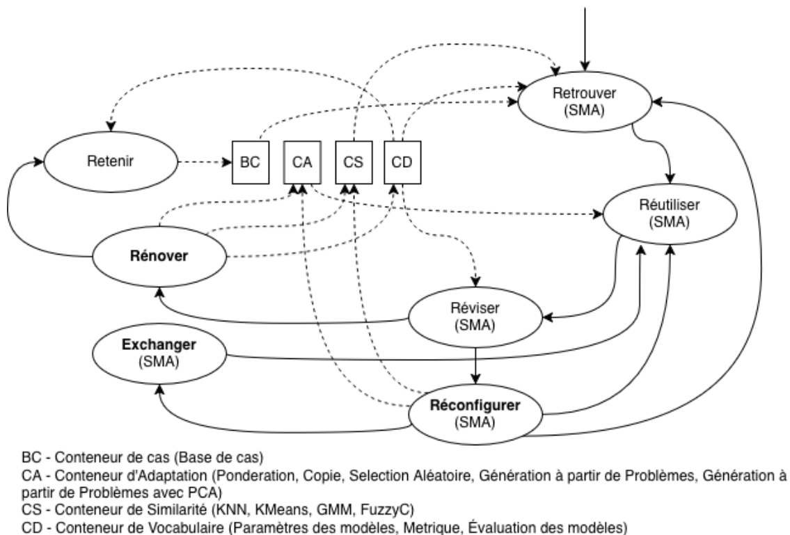
FIGURE 6.8 – Deux cycles du système ESCBR-SMA proposé.
