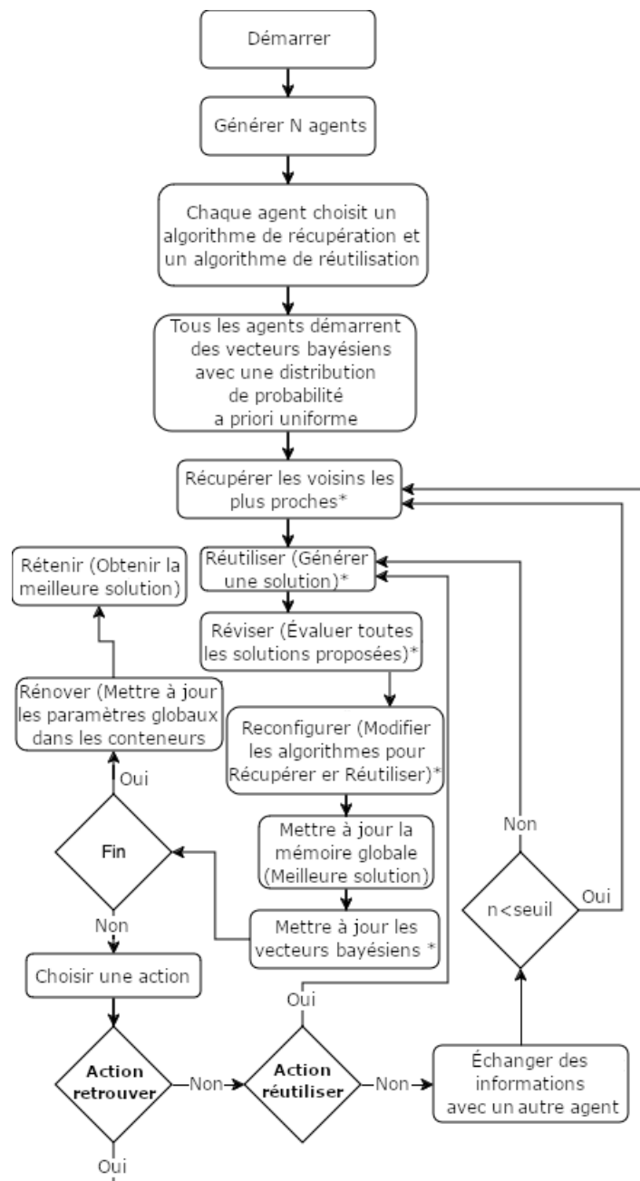
FIGURE 6.9 – Flux du Stacking du RàPC (* : tâche effectuée par chaque agent).
