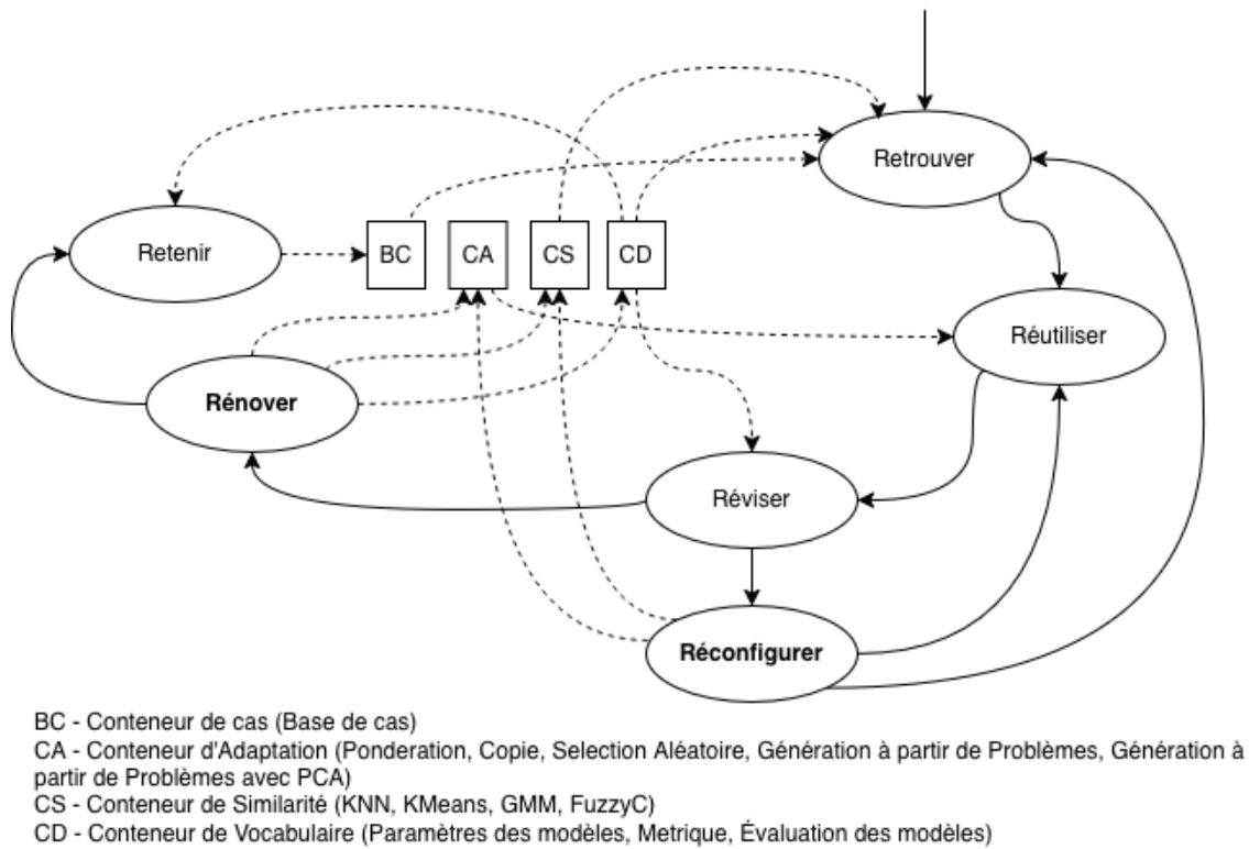
FIGURE 6.1 – Les deux cycles proposés pour le RàPC.
