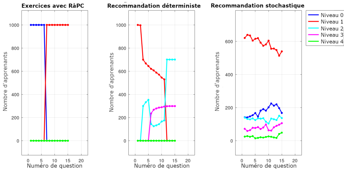
FIGURE 7.3 – Niveaux de complexité des questions posées aux apprenants par les trois systèmes testés lors de la deuxième séance. À gauche - RàPC, au centre - recommandation déterministe (DM), à droite - moyenne de 100 exécutions de recommandation stochastique (SM).
