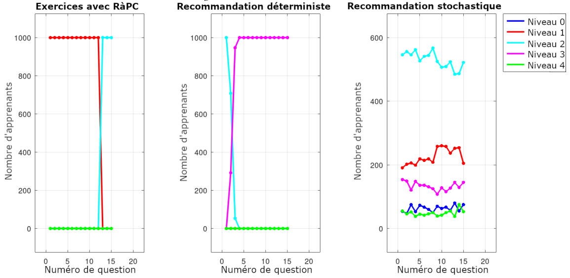
FIGURE 7.4 – Niveaux de complexité des questions posées aux apprenants par les trois systèmes testés lors de la troisième séance. À gauche - RàPC, au centre - recommandation déterministe (DM), à droite - moyenne de 100 exécutions de recommandation stochastique (SM).
