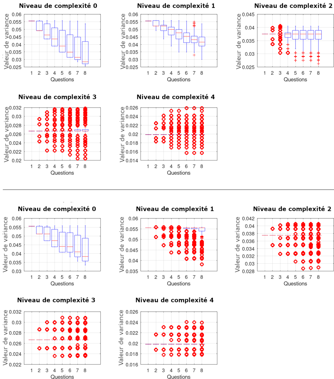
FIGURE 7.16 – Variance pour la distribution de probabilité bêta et tous les niveaux de complexité (en haut : processus d'apprentissage statique. En bas : processus d'apprentissage dynamique avec processus de Hawkes).
