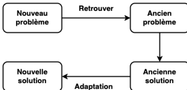
FIGURE 2.4 – Principe de réutilisation dans le RàPC (traduit de Richter et Weber (2013)).
