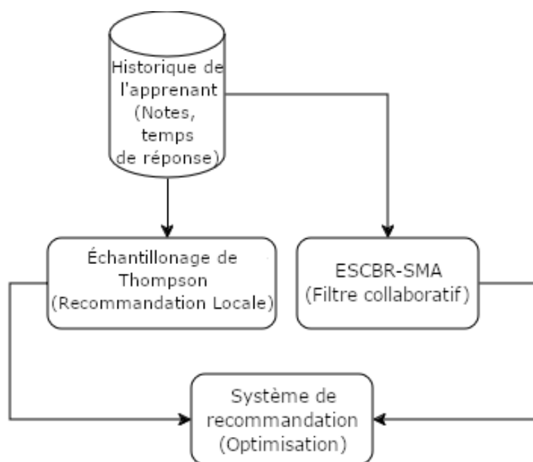
FIGURE 7.7 – Schéma de l'architecture du modèle proposé
