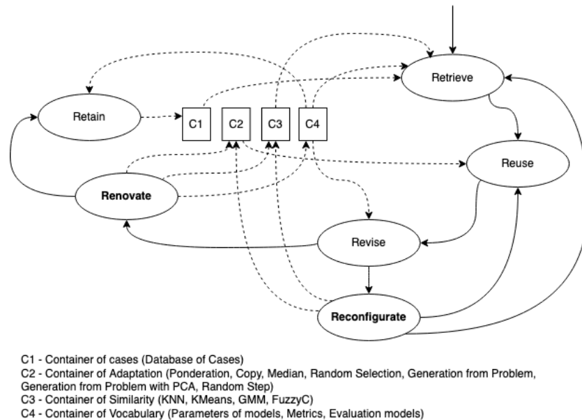
FIGURE 6.1 – Les deux cycles proposés pour le RàPC
