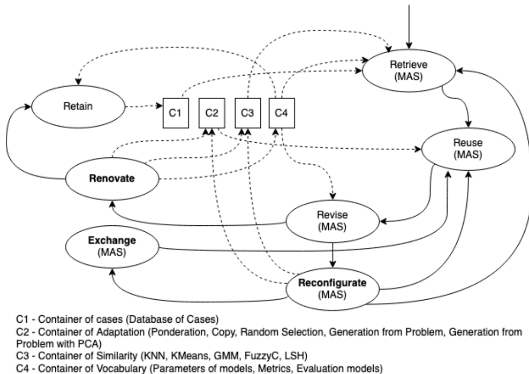
FIGURE 6.8 – Deux cycles du système ESCBR-SMA proposé
