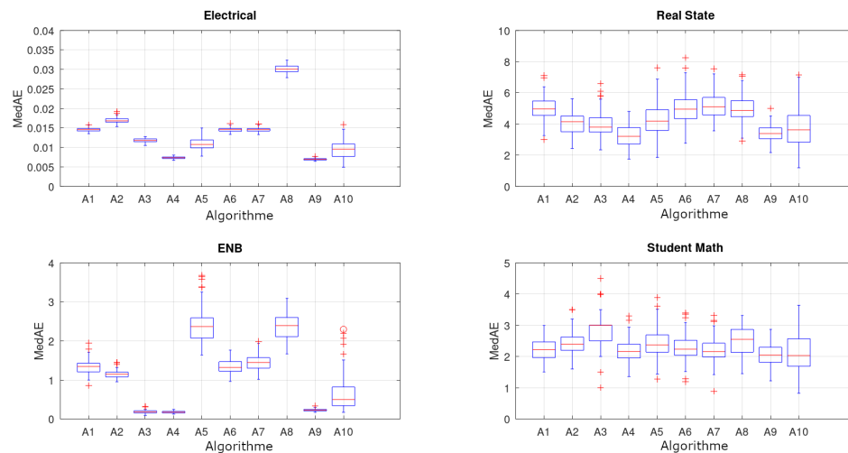
FIGURE 6.7 – Résultats de la métrique MAE ( Median Absolute Error ) pour les dix algorithmes et quatre bases de données représentatives
