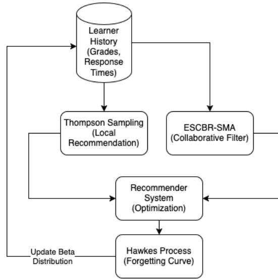
FIGURE 7.12 – Architecture de modèle proposé avec Hawkes
