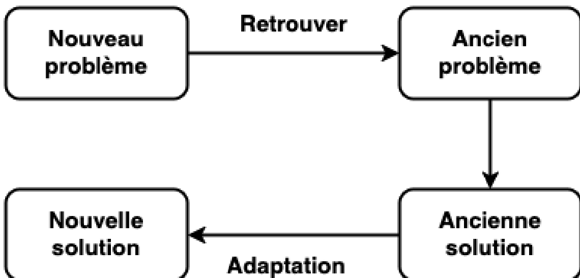
FIGURE 2.4 – Principe de réutilisation dans le RàPC ([Richter and Weber, 2013])
