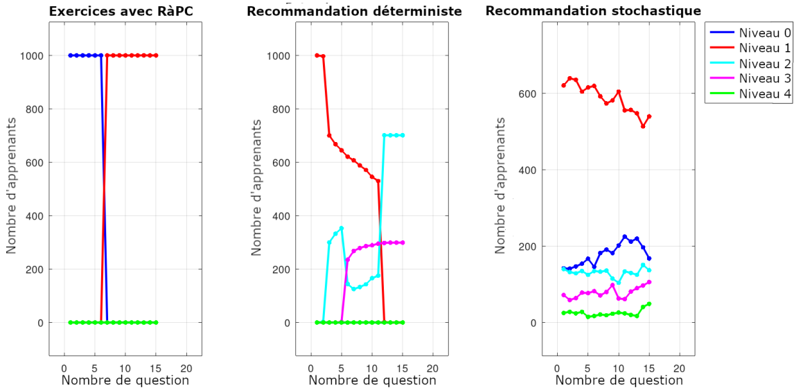
FIGURE 7.3 – Résultats pour le deuxième Test
