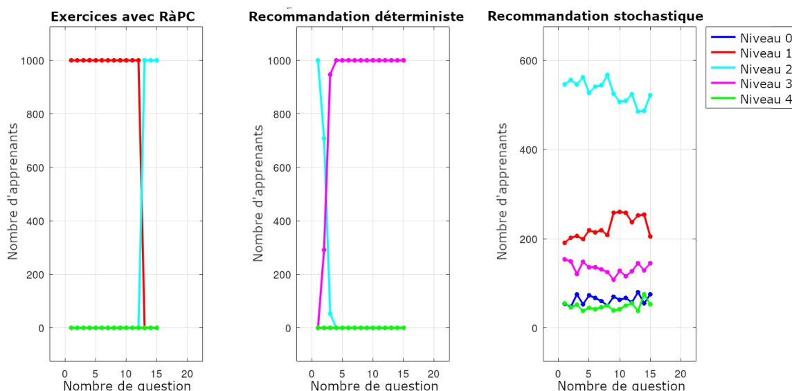
FIGURE 7.4 – Résultats pour le troisième Test
