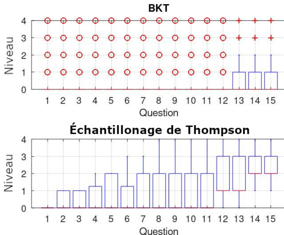
FIGURE 7.10 – Comparaison de l'évolution des niveaux entre les algorithmes BKT et TS
