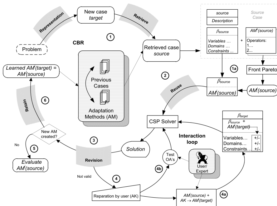
FIGURE 4.1 – Cycle du RàPC modifié. ([Roldan Reyes et al., 2015])
