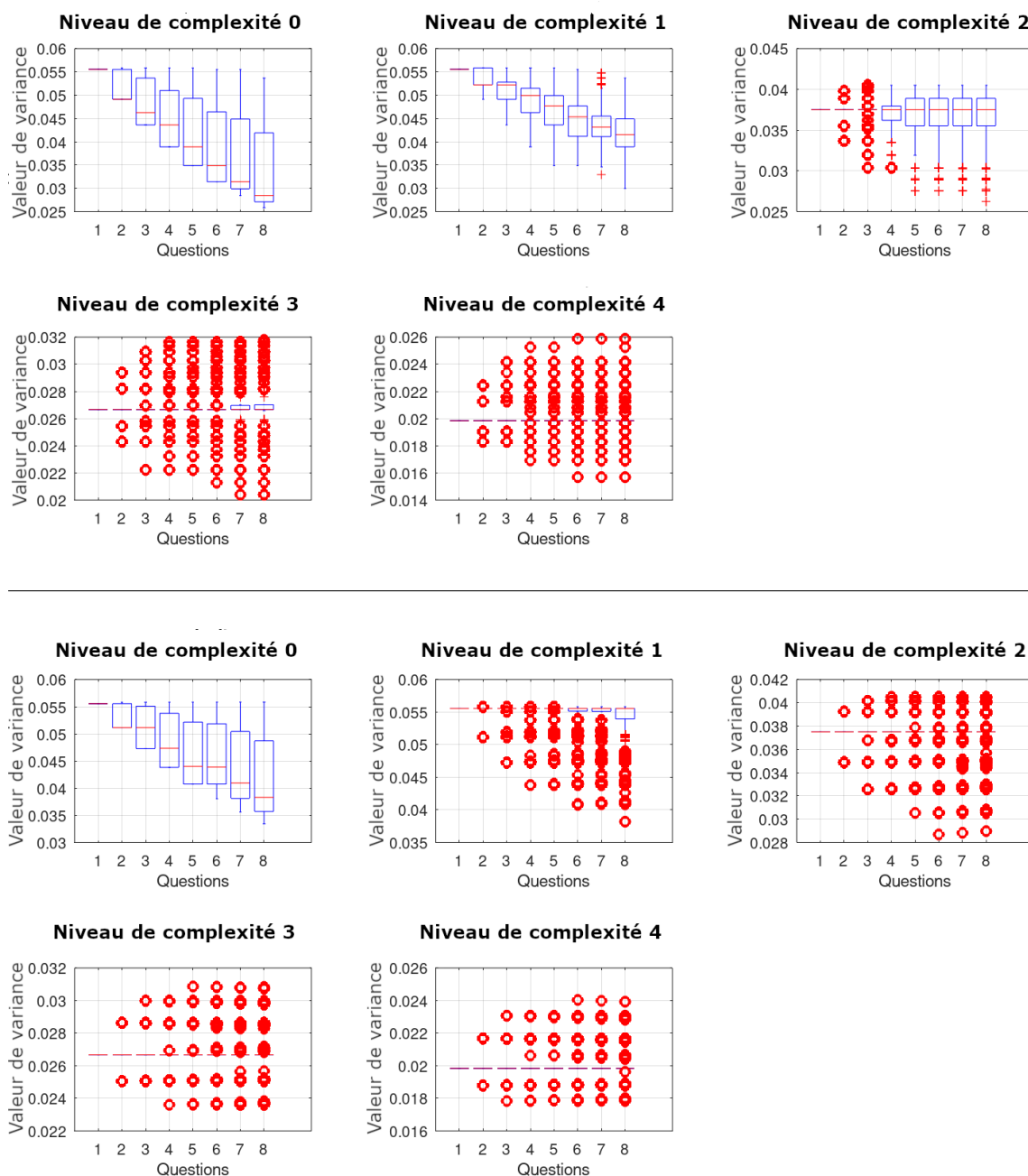
FIGURE 7.14 – Évolution de la variance pour la distribution de probabilité bêta et tous les niveaux de complexité (en haut : processus d'apprentissage statique. En bas : processus d'apprentissage dynamique avec processus de Hawkes)
