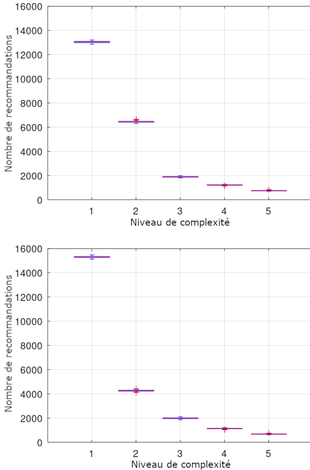
FIGURE 7.13 – Nombre de recommandations par niveau de complexité (à gauche processus d'apprentissage statique, à droite processus d'apprentissage dynamique avec processus de Hawkes)
