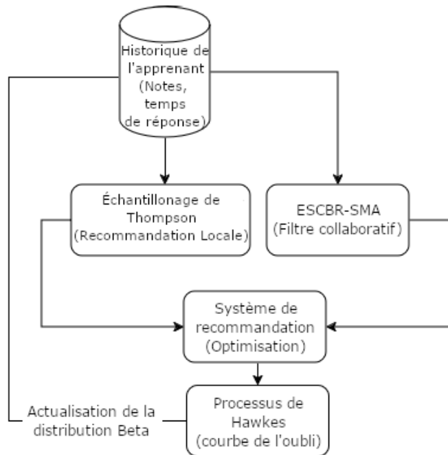
FIGURE 7.12 – Architecture de modèle proposé avec Hawkes
