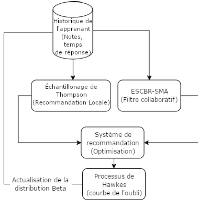
FIGURE 7.12 – Organisation des modules TS, ESCBR-SMA et processus de Hawkes.
