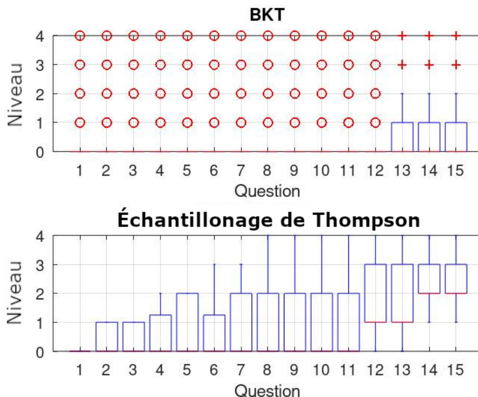
FIGURE 7.10 – Comparaison de l'évolution des niveaux entre les systèmes de recommandation fondés sur BKT et TS
