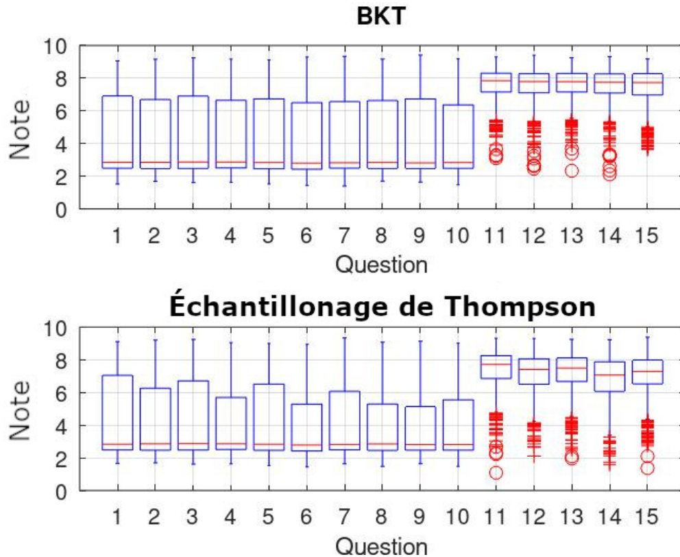
FIGURE 7.9 – Comparaison de l'évolution des notes entre les systèmes fondés sur TS et BKT.
